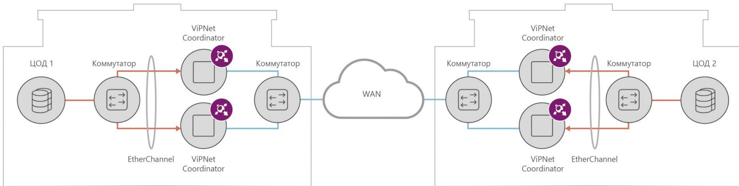
ЛВС Эластичного ЦОД
